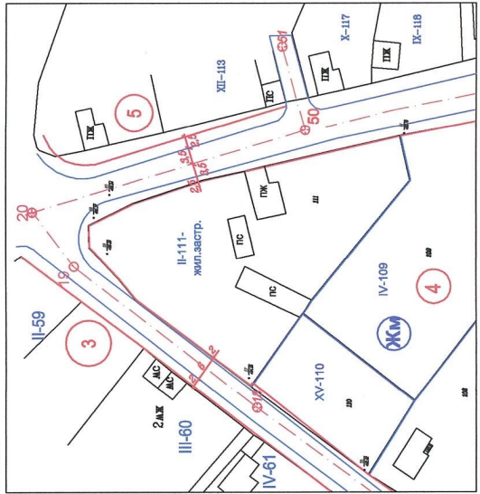
ПЛАН за РЕГУЛАЦИЯ на УПИ II-111-ЖИЛ.застр., кв.4 по плана на с.Смилец, Община Стрелча, обл.Пазарджик М 1:1000
