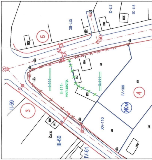
ИЗМЕНЕНИЕ на ПЛАН за РЕГУЛАЦИЯ на УПИ I-111 и УПИ II-111, кв.4 по плана на с.Смилец, Община Стрелча, обл.Пазарджик М 1:1000
