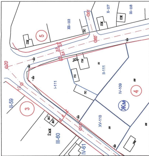
КОМБИНИРАНА ИЗВАДКА от дворична и улчна регулация за УПИ I-111 и УПИ II-111, кв.4 по плана на с.Смилец, Община Стрелча, обл.Пазарджик М 1:1000
